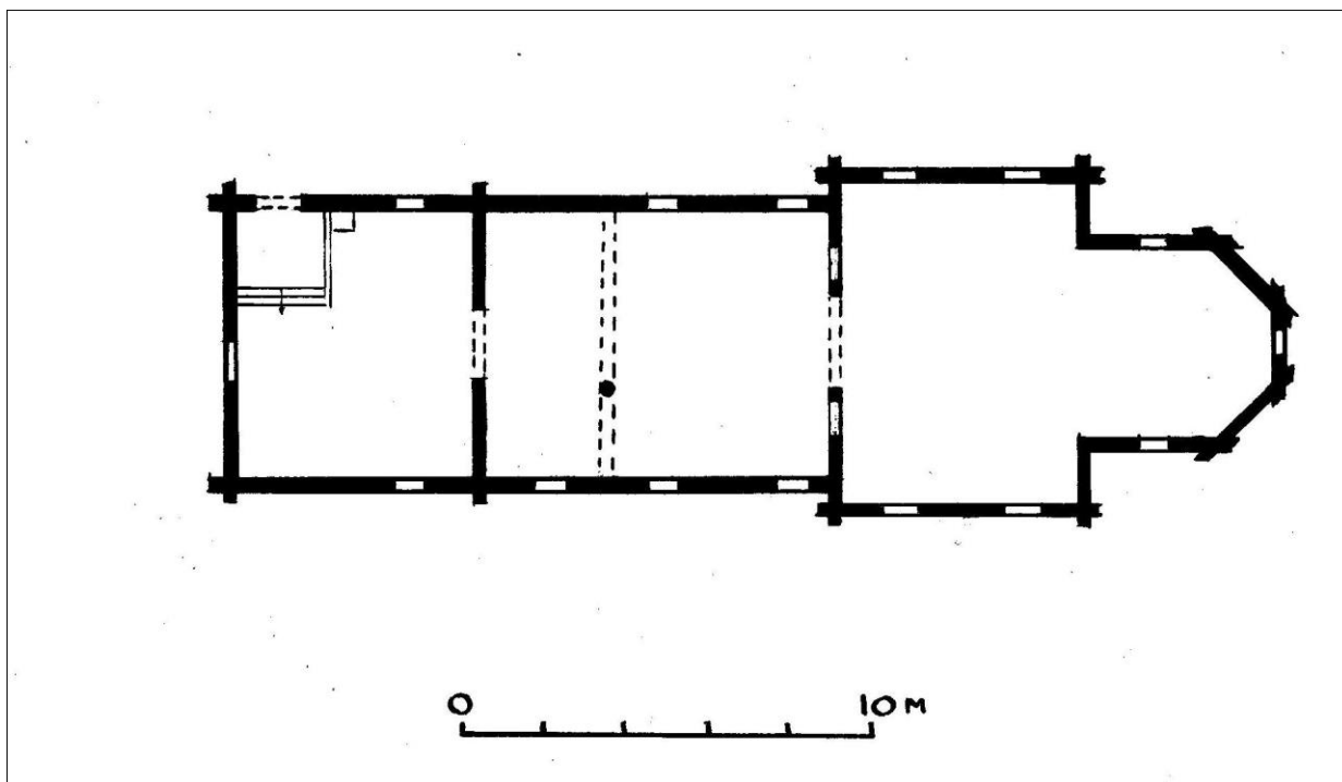
Рис. 7в. Корбала. Церковь Параскевы Пятницы. План. Обмер 1971 г.
